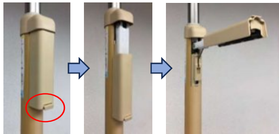
ロックボタン 下にスライド 長いストロークで操作しやすい
