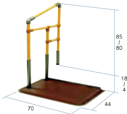
あがりかまち用 たちあっぷミニ片手すり
