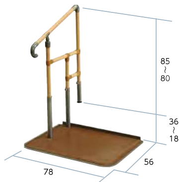
あがりかまち用 たちあっぷ片手すり
