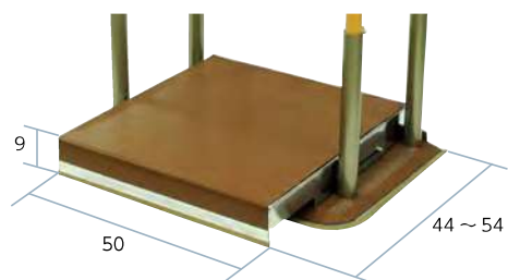
たちあっぷミニスライドベース
