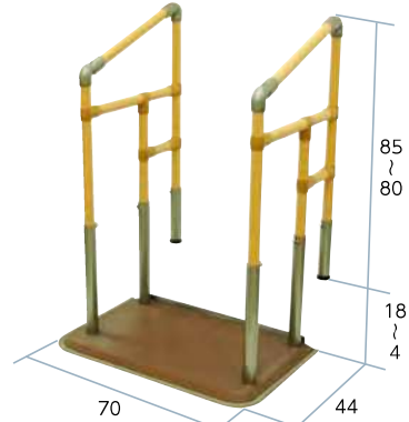
あがりかまち用 たちあっぷミニ両手すり
