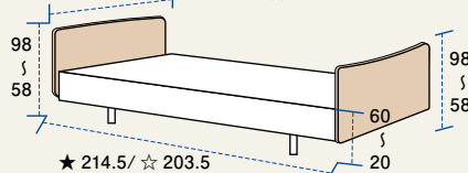
ベッド寸法図 (cm)
