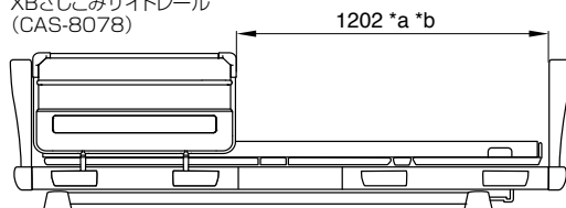
XBさしこみサイドレール (CAS-8078)
