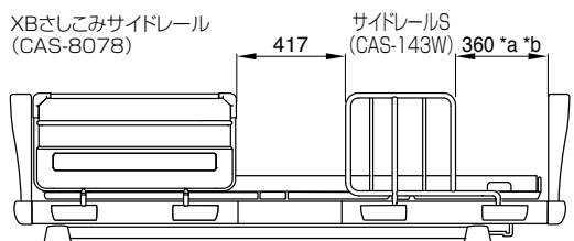
XBさしこみサイドレール (CAS-8078)
