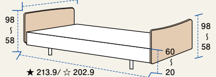
ベッド寸法図 (cm)
