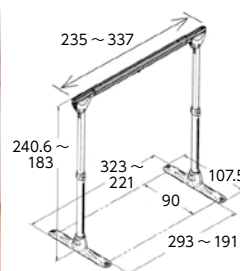
寸法図 (cm)
