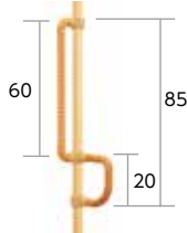
ベースポジ BPZ ツイン手すり W+D
