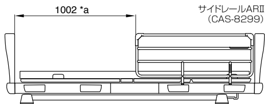
サイドレールARII (CAS-8299)
